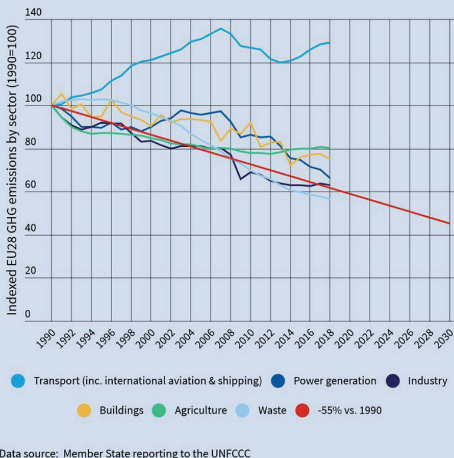
Fig.1: Trend delle emissioni di CO 2 per settore. Fonte: UNFCCC, 2018
