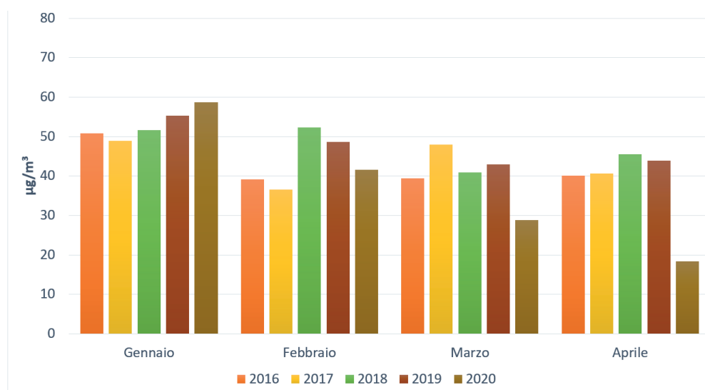
Figura 11 – Napoli: Media mensile del \text{NO}_2 delle stazioni di traffico nei mesi di Gennaio, Febbraio, Marzo ed Aprile per le annualità 2016-2020
