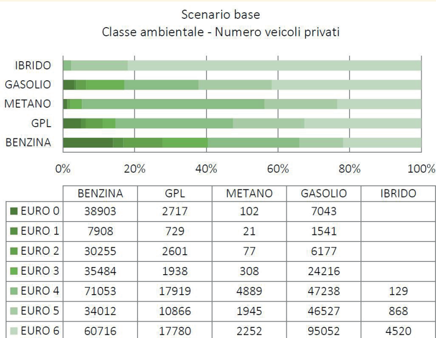
Figura 2. Ripartizione per tecnologia e classe ambientale veicoli privati - Comune Torino
