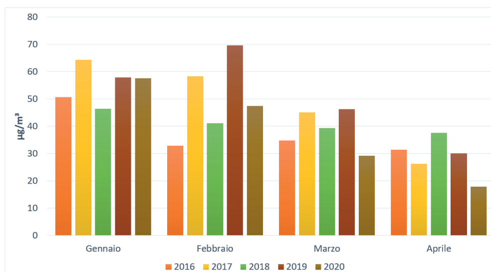
Figura 5 – Milano: Media mensile del \text{NO}_2 delle stazioni di traffico nei mesi di Gennaio, Febbraio, Marzo ed Aprile per le annualità 2016-2020
