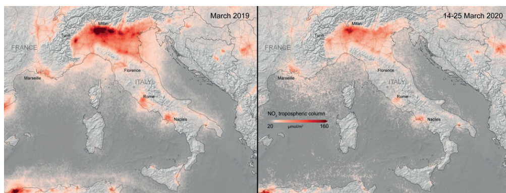
Figura 1 - Immagine elaborata da dati satellitari di Copernicus Sentinel-5P, che mostrano la media delle concentrazioni di biossido di azoto dal 14 al 25 Marzo 2020, confrontate con la media mensile delle concentrazioni di Marzo 2019
