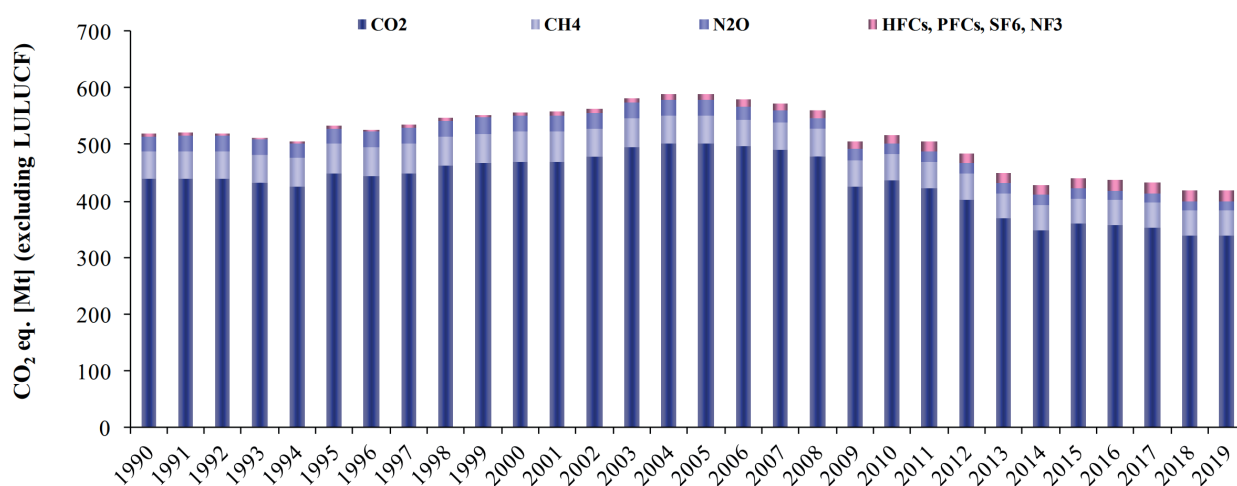
Figura 1 Andamento delle emissioni dei gas serra dal 1990 al 2019 (senza LULUCF) (ISPRA, 2021)
