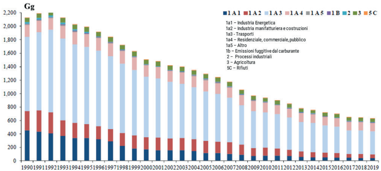
Figura 2 - Trend delle emissioni di NO x per settore 1990-2019 (ISPRA, 2021)
